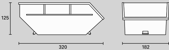
Absetzmulde 5,5m 3
