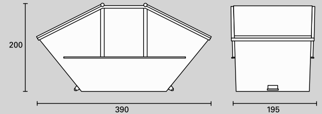
Absetzmulde mit Deckel 10m 3
