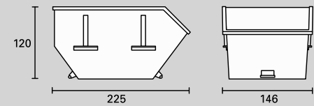
Citymulde 3m 3
