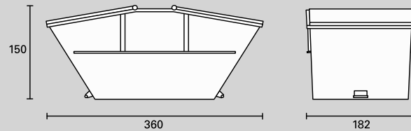
Absetzmulde mit Deckel 7m 3
