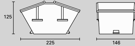
Citymulde mit Deckel 3m 3
