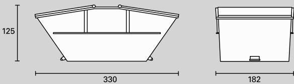
Absetzmulde mit Deckel 5m 3
