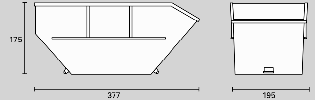
Absetzmulde 10m 3
