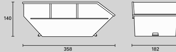
Absetzmulde 7m 3
