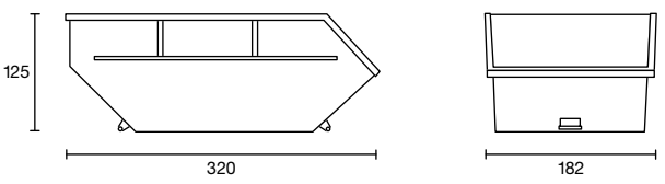
Absetzmulde 5 m³
