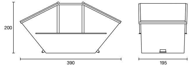
Absetzmulde mit Deckel 10 m³
