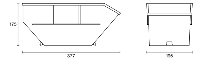
Absetzmulde 10 m³
