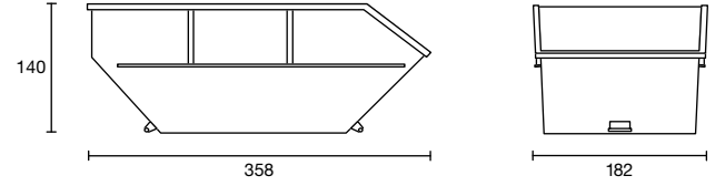
Absetzmulde 7 m³
