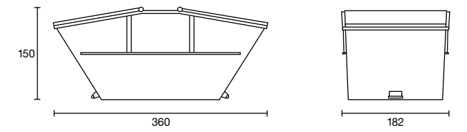
Absetzmulde mit Deckel 7 m³
