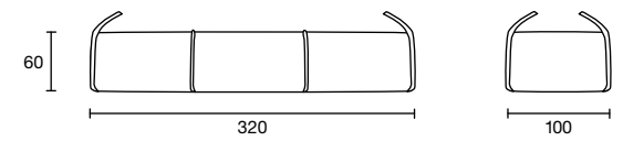
Asbest-BIG BAG 2,2 m³
