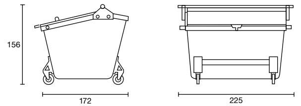
Umlerer 3 cbm
