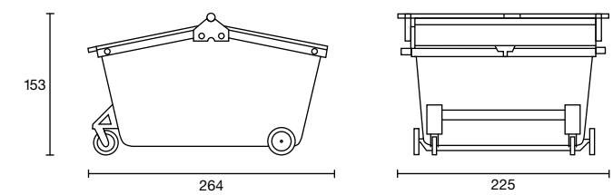
Umlerer 5 cbm
