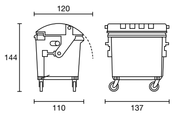
Umlerer 1100 ltr
