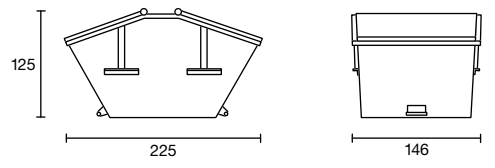
Citymulde mit Deckel 3 m³
