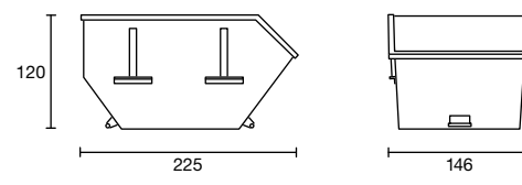
Citymulde 3 m³
