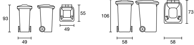
Umlerer 120 ltr
