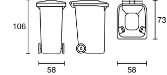
Umlerer 240 ltr
